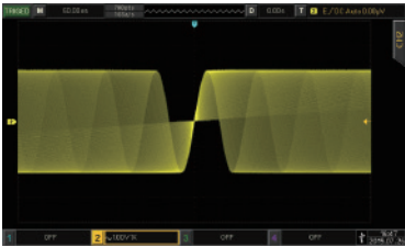
3 高达83,000wfms/s波形捕获率, 大大提高了捕获及低概率事件的能力, 可更直观的观察信号抖动和毛刺
